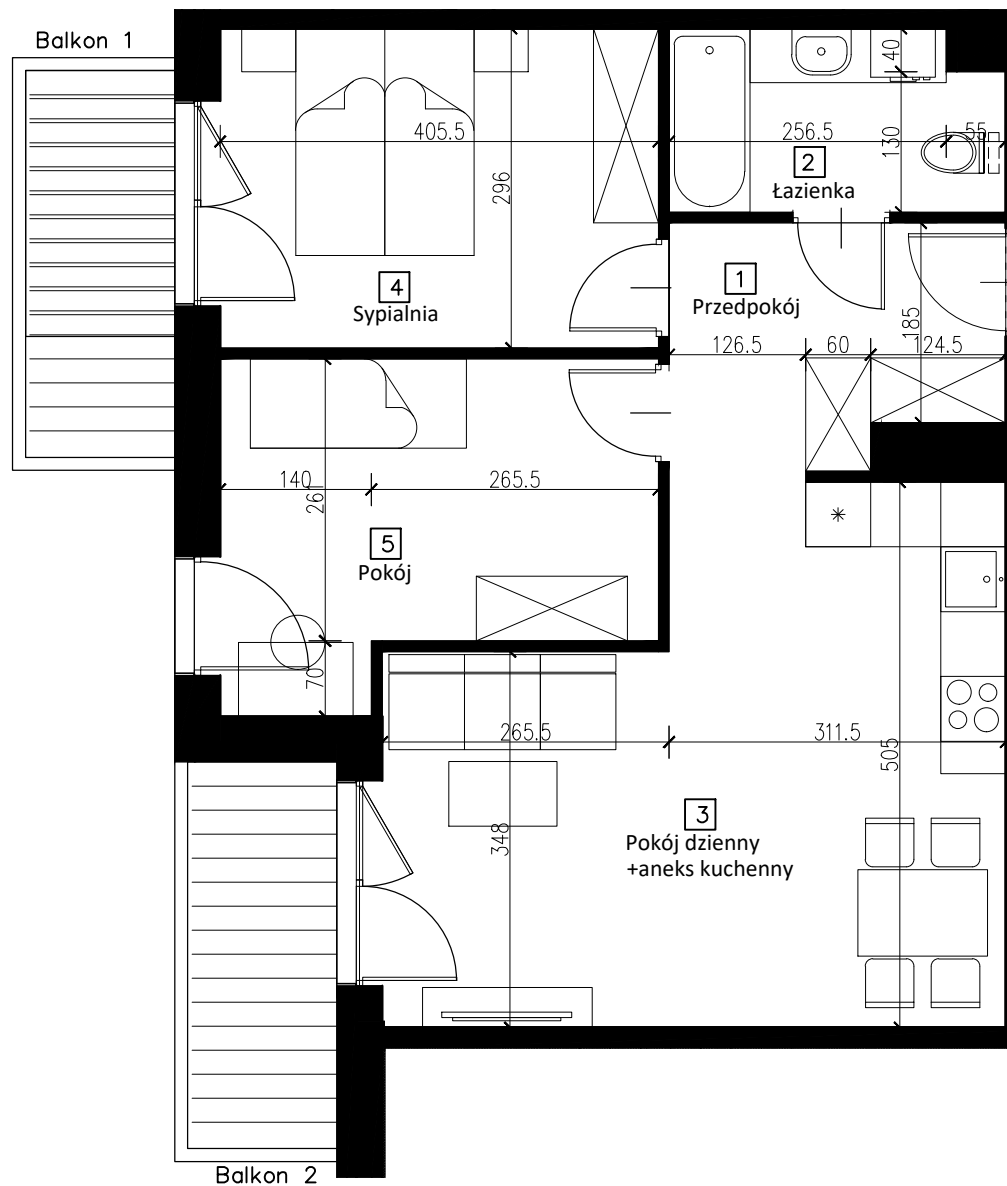
PIĘTRO II
